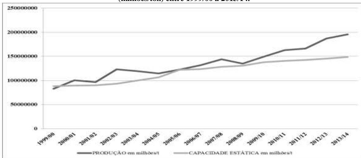
Figura 1 – Evolução da produção de grãos (milhões/ton) e evolução da capacidade de armazenamento (milhões/ton) entre 1999/00 à 2013/14.
